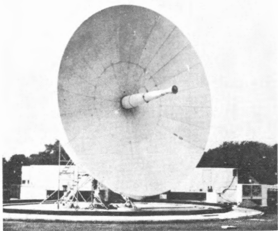
AN/MSC-46 ANTENNA
