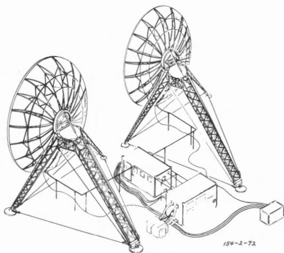
AN/TRC-132A
