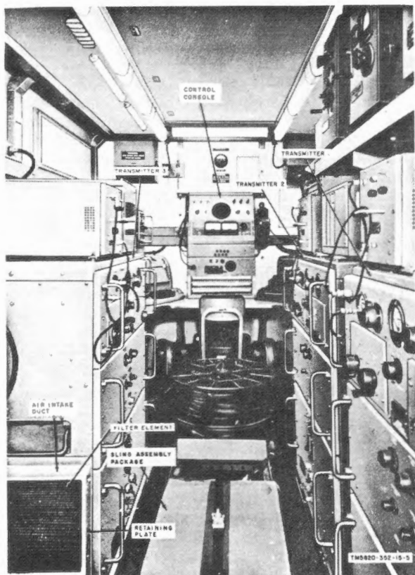
AN/MRT-9
