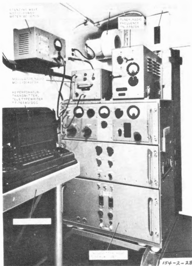
AN/GRC-26D
