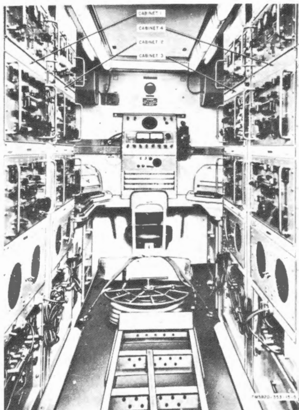
AN/MRR-8
