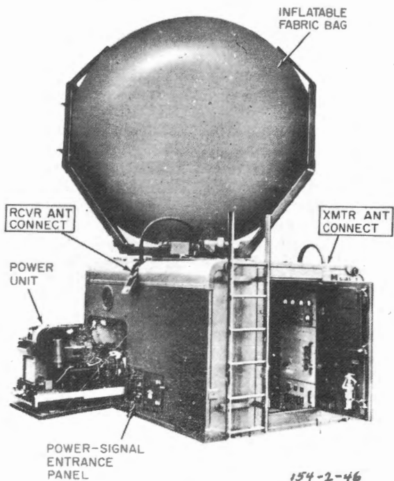
AN/TRC-80
