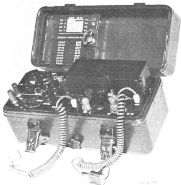
AN/PRC-64
